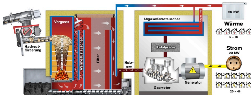
Schema cogenerazione calore-legno Hargassner
