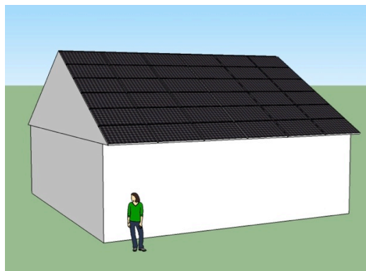
Casa unifamiliare 140 m 2 SRE, fabbisogno energetico 12.000 kWh/anno, ad es. con pompa di calore e mobilità elettrica, 10 kWp PV = 714% del minimo, copre >70% del consumo annuo, autoconsumo 40-60%
