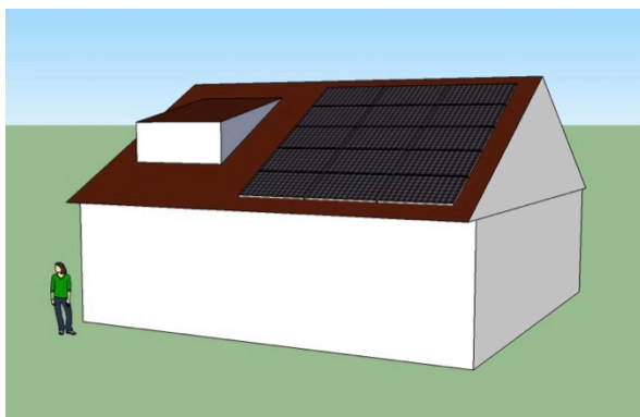
Casa unifamiliare 140 m 2 SRE, fabbisogno energetico 4000 kWh/anno, ad es. con riscaldamento a pellet di legno e resistenza elettrica WW 4 kWp PV = 285% del minimo, copre >80% del consumo annuo, autoconsumo 20-40%
